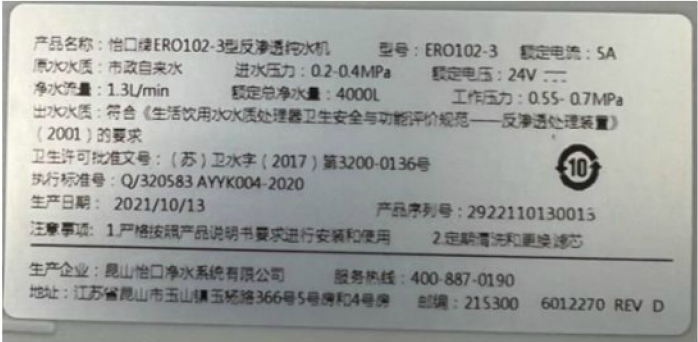
ERO102-3（铭牌）
